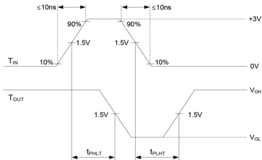
图1. t_{\text{PHL}} 和 t_{\text{PLH}} 波形
