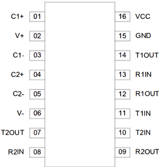
SOP -16 PKG
