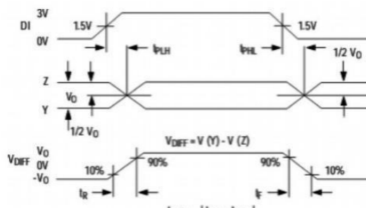
图 8 驱动传输延时
