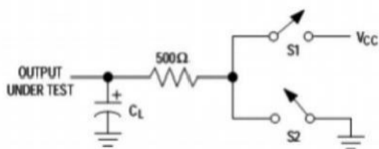
图6驱动时间测试电路
