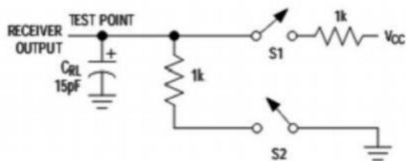
图4接收时间测试电路
