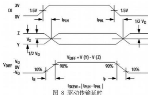
图 8 驱动传输延时
