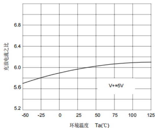
充放电电流之比与温度关系
