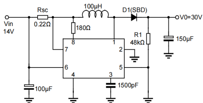
图1 升压变换器
