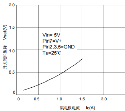
开关饱和压降与集电极电流关系
