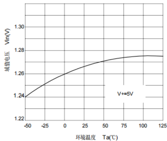
域值电压与温度关系
