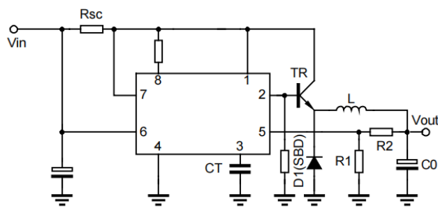
图4 降压变换器（大电流）
