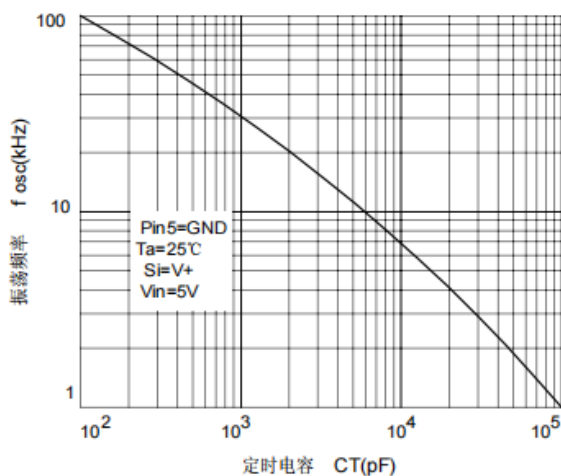
振荡频率与定时电容关系
