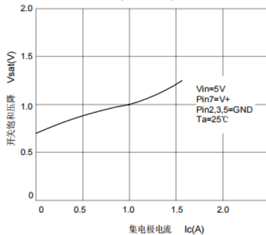
开关饱和压降与集电极电流关系 (达林顿方式)
