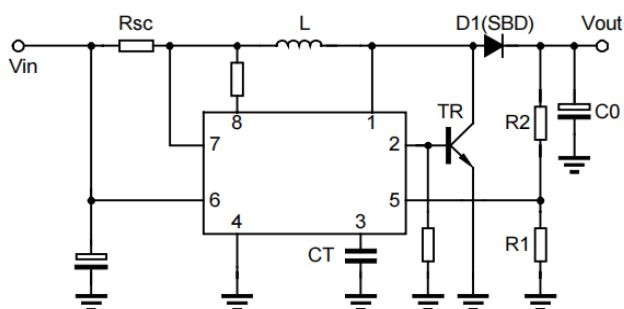
图3 升压变换器（大电流）
