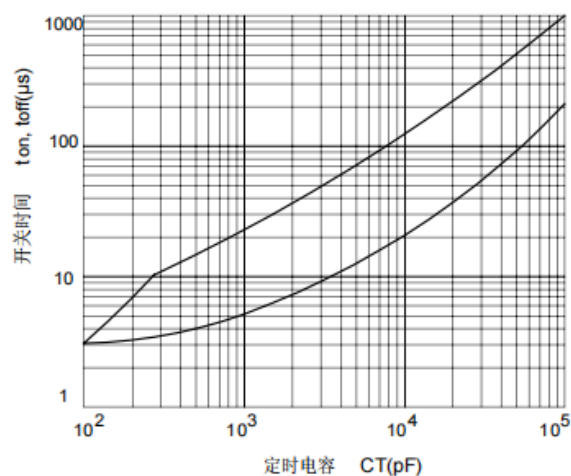
开关时间与定时电容关系
