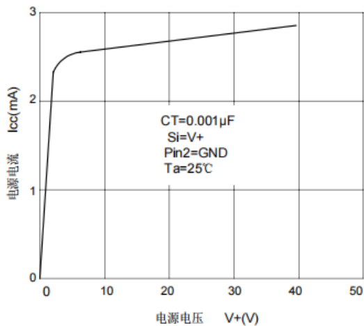
电源电流与电源电压关系
