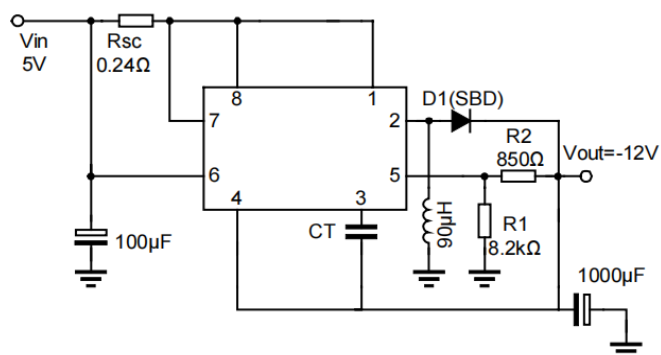
图5 反向变换器
